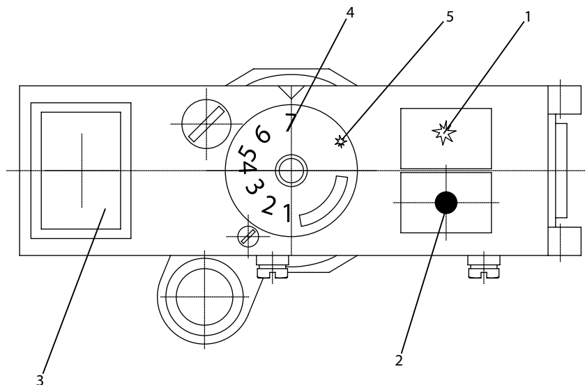
Рисунок 2 — Блок газовый
